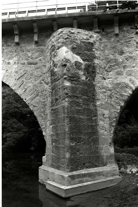
Détail de la pile centrale du pont Fig. 3 (JPD, 6. 8. 1992)
